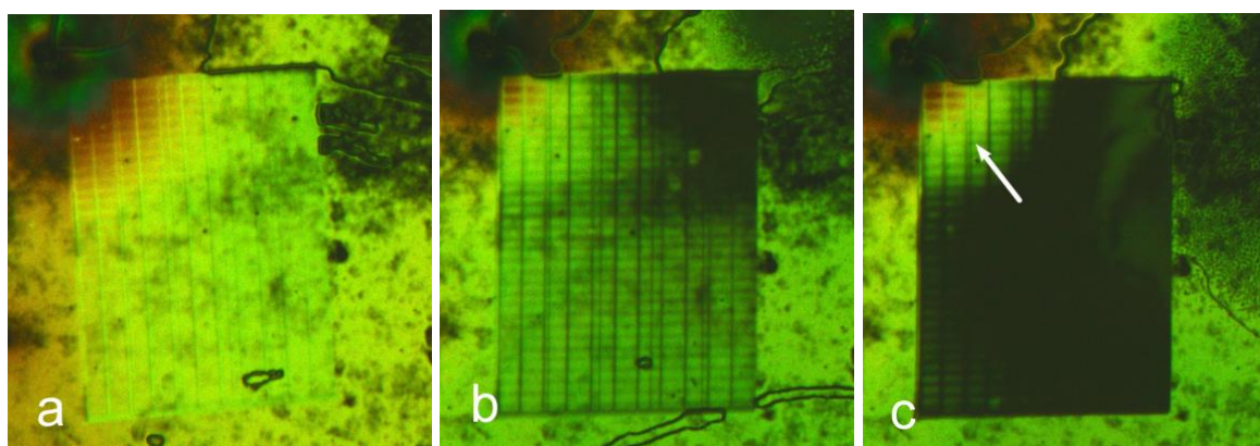
Рис. 4. Реакция нематика на пары диметилформамида над наноразмерной углеродной решеткой. а – Исходная ориентация нематика над решеткой. б – Гомеотропная ориентация нематика над полосами решетки. с – Гомеотропная ориентация нематика над всей поверхностью углеродной решетки
