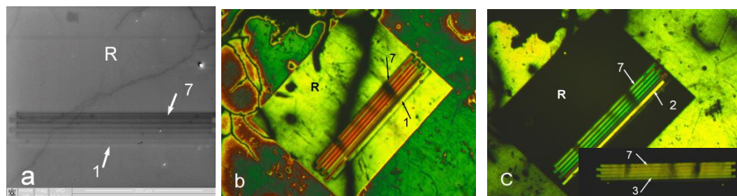
Рис. 2. Переход нематика из наклонного в гомеотропное состояние ориентации над углеродными плёнками. а – РЭМ изображение углеродных плёнок (1–7) полученных электронным лучом в камере микроскопа. R – полный электронный растр участка. Растр каждой индивидуальной углеродной плёнки нагара 500 \times 10 \mu\text{m} . Ток напыления 37 нА. Время напыления плёнок, s: 1–1, 2–10, 3–20, 7–60. б – Поляризационное изображение слоя нематика сразу после нанесения на растр R с углеродными плёнками. с – Тот-же образец с жидким кристаллом через 2 суток.
