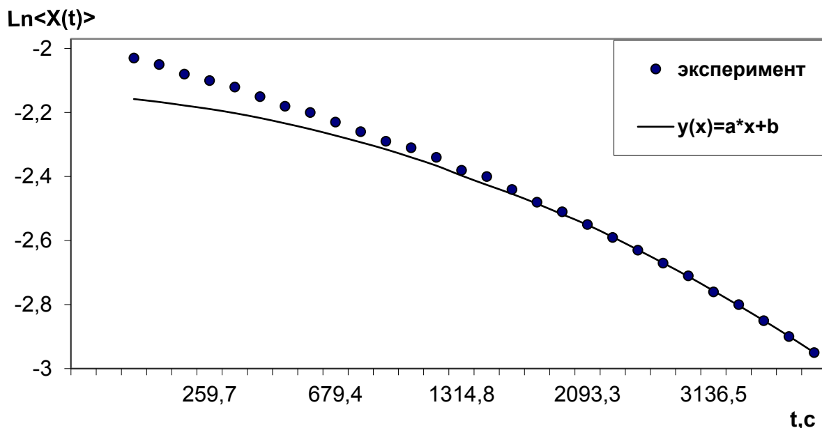
Рис. 2 Сравнение экспериментальных значений, измерения логарифма средней концентрации со временем, с расчётными Fig. 2 Comparison of experimental values, measurement of the logarithm of mean concentration with time, with calculated
