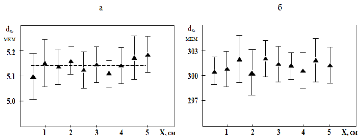
Рис. 4. Экспериментальное определение проекций вектора смещения при смещении объекта как целого вдоль оси X на величину: а – d_0 = 5 мкм; б – d_0 = 300 мкм
