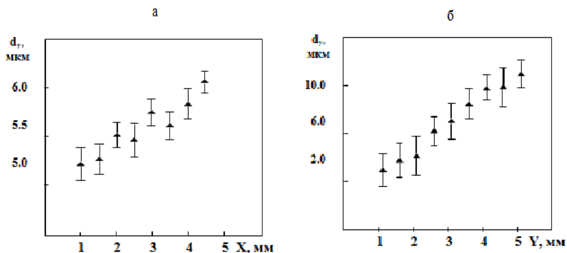
Рис. 5. Изменение проекций вектора смещения поверхности нагруженного объекта вдоль направлений: а – X; б – Y
