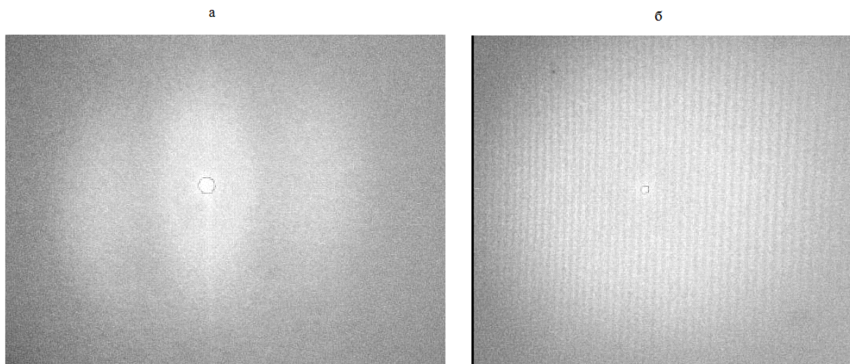
Рис. 2. Спеклограммы при критической величине вектора смещения: а – при d = 12 \text{ мкм} ; б – при d = 180 \text{ мкм} . На второй фотографии смещение порядка 180 \text{ мкм} Fig. 2. Specklegram when the critical value of the displacement vector: а – d = 12 \text{ }\mu\text{m} ; б – d = 180 \text{ }\mu\text{m} In the second photo, the displacement is about 180 \text{ }\mu\text{m}
