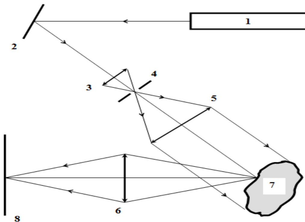
Рис. 3. Оптическая схема записи спеклограмм: 1– лазер ЛГН-215, \lambda = 0,6328 \text{ мкм} ; 2 – поворотное зеркало; 3 – микрообъектив ( 10\times ); 4 – точечная диафрагма ( 30 \text{ мкм} ); 5 – линза коллиматора; 6 – объектив; 7 – диффузный объект; 8 – фотопластинка Fig. 3. Optical scheme of recording specklegrams: 1– laser LGN-215, \lambda = 0,6328 \text{ }\mu\text{m} ; 2 – rotary mirror; 3 – micro lens ( 10\times ); 4 – point aperture ( 30 \text{ }\mu\text{m} ); 5 – collimator lens; 6 – lens; 7 – diffuse object; 8 – photographic plate
