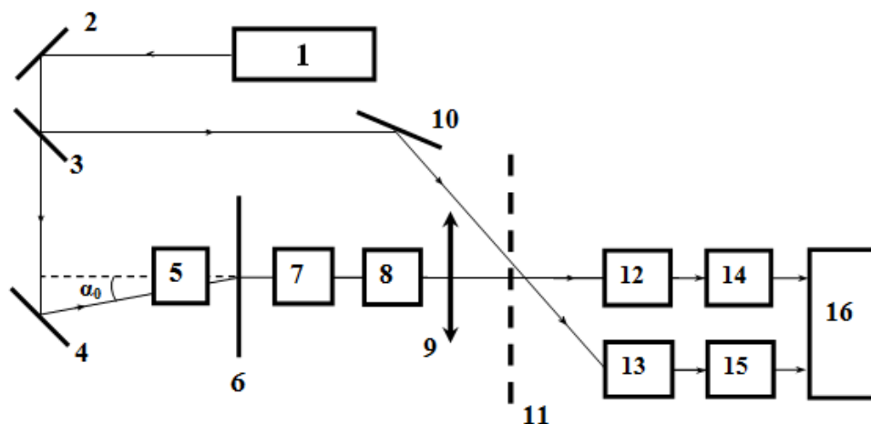
Рис. 1. Принципиальная схема устройства обработки спеклограмм
