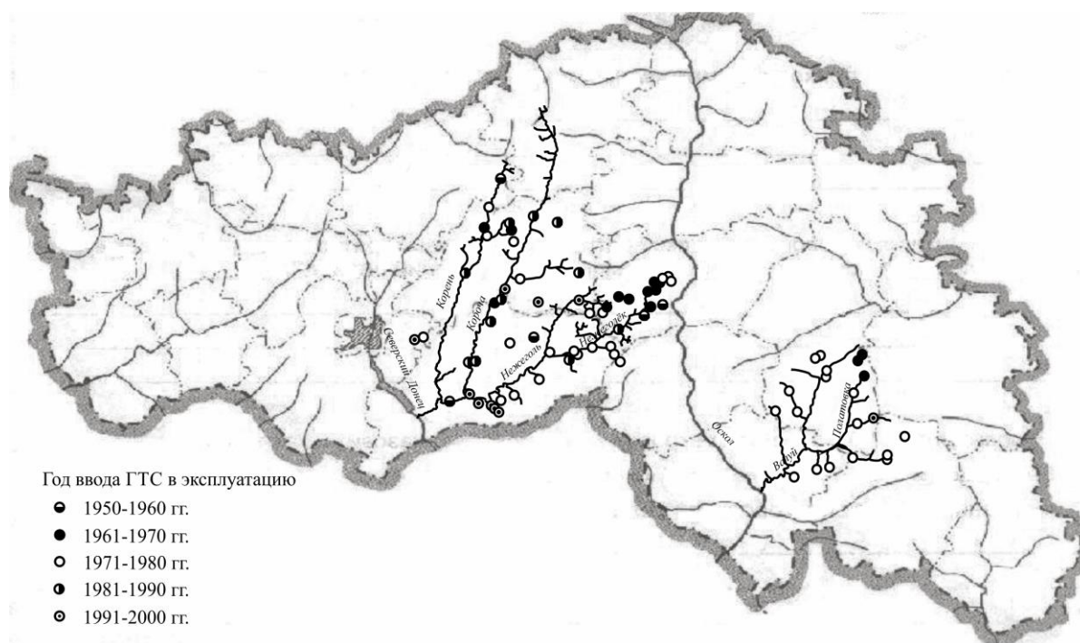
Рис. 8. Хронология ввода в эксплуатацию ГТС на р. Нежеголь и р. Валуй и их притоках Fig. 8. Chronology of commissioning of the GTS on the Nezhgol river and the Valui river and their tributaries
